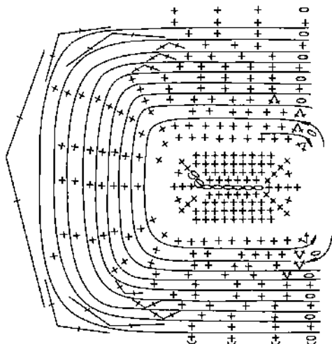
Схема вязания пинеток-пуантов
