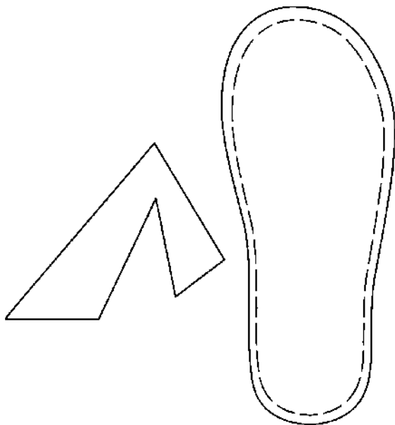
Выкройка шлепанцев «Уголки»
