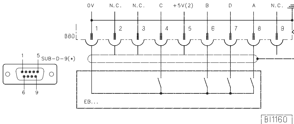
EB.. Actuator
