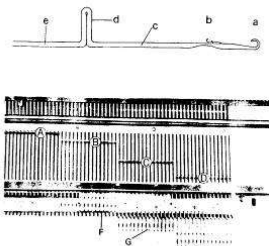
Игольница и положение игл в ней
