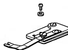
Separator 159321-101
