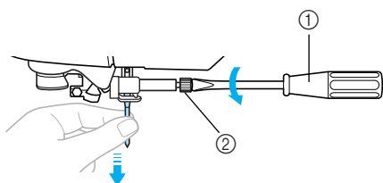
① Отвертка ② Винт иглодержателя
